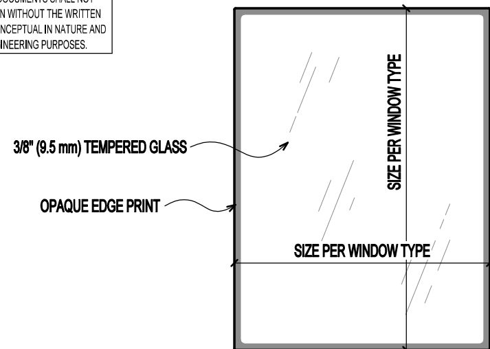
GLASS PANEL DETAIL SCALE: N.T.S.
